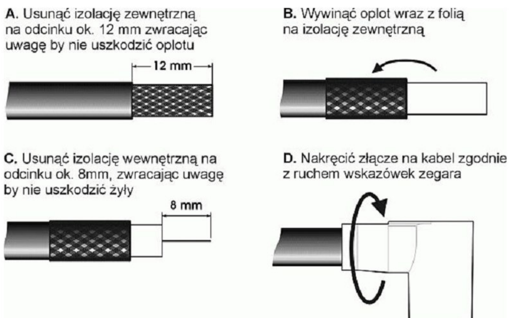
Rys.1. Sposób montażu złącz serii WKS, WKW, WKG na kablu koncentrycznym.
