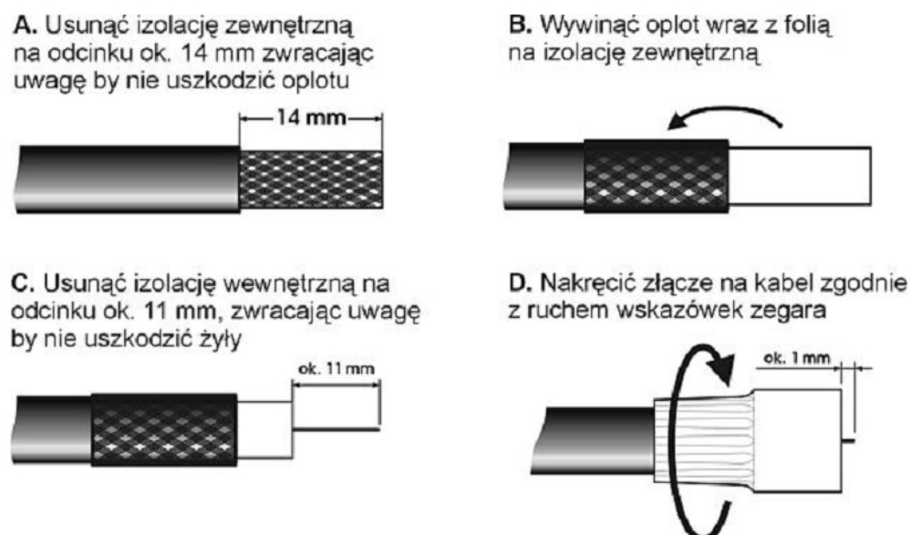
Rys.2. Sposób montażu złącz serii WPS, WPW, WPG na kablu koncentrycznym.
